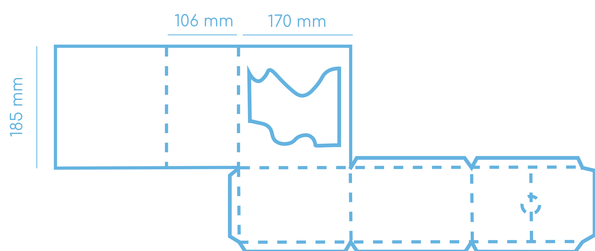
vnější rozložení krabice
