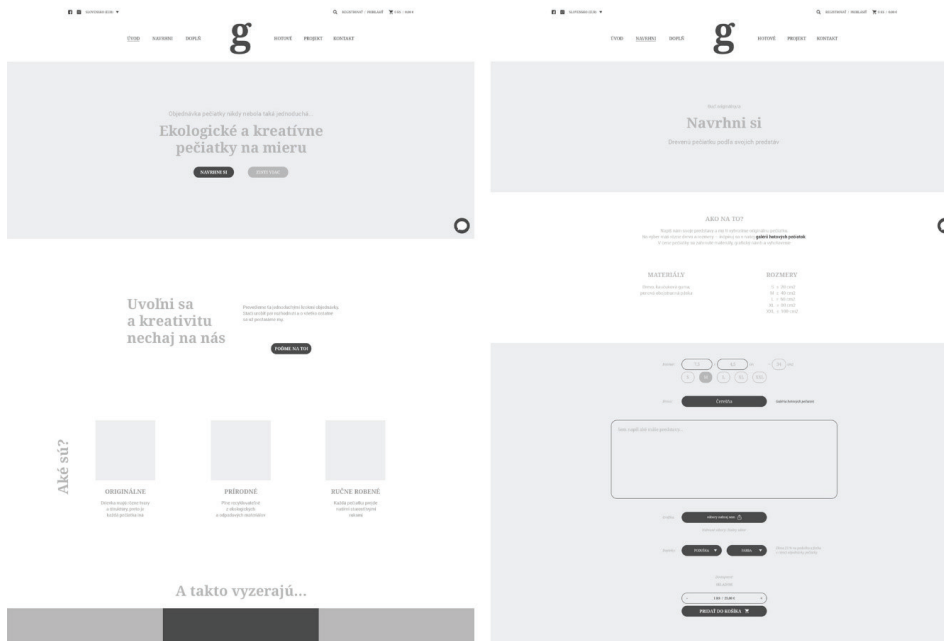
Obr. 28. Wireframe úvodnej stránky a podstránky
