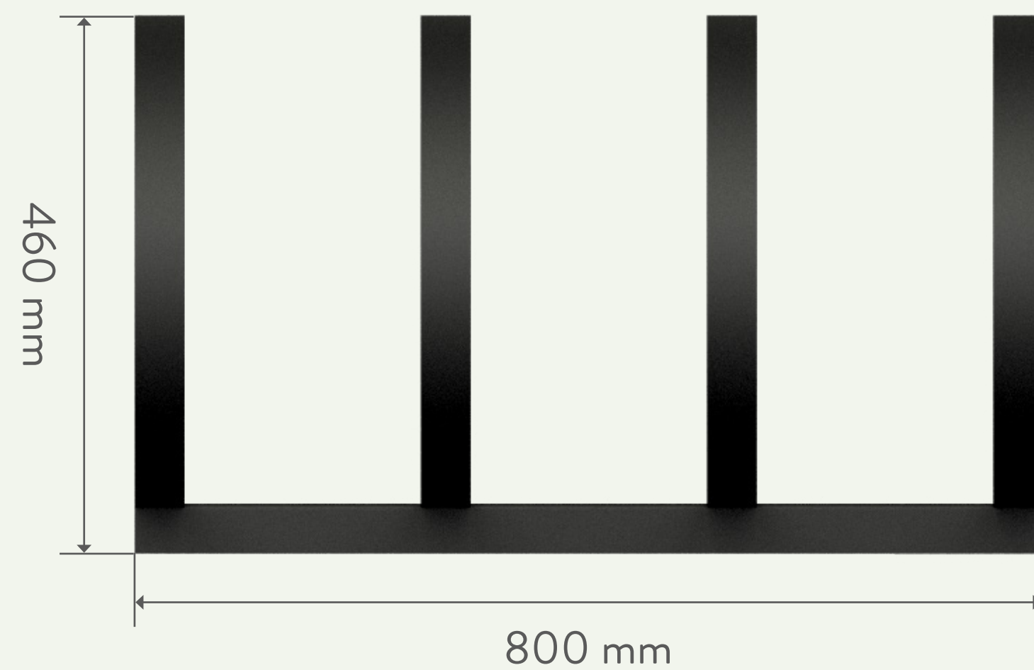
čelný pohľad:
