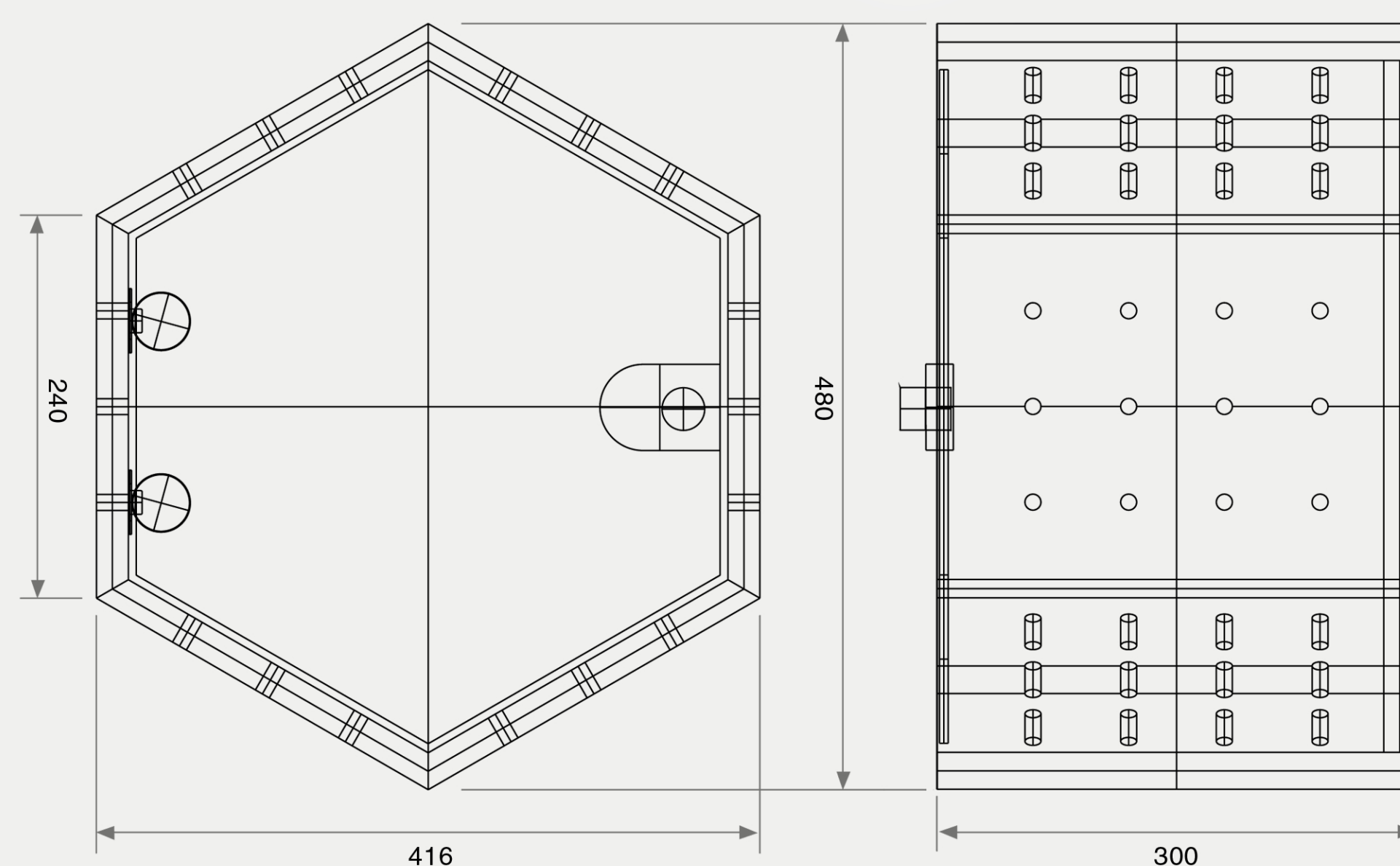
spojování pomocí kolíků
