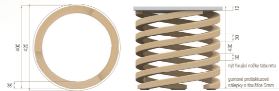
rozměry taburetu v mm
